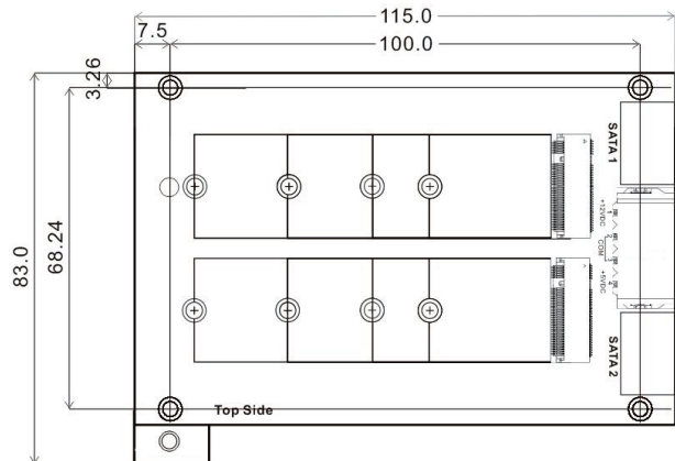
外型尺寸 (單位:mm)
