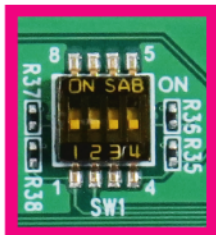
EEPROM : 24AA256T SETUP
