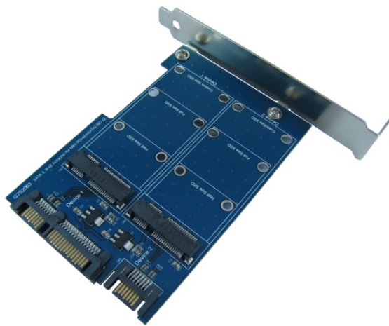
Mini PCI-e (mSATA) Custom Size
