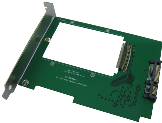
CB945MB 轉接卡
