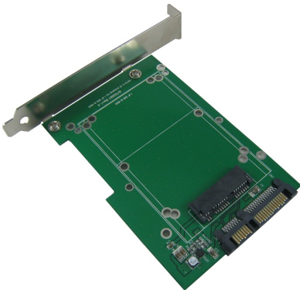
AD962FB 轉接卡
