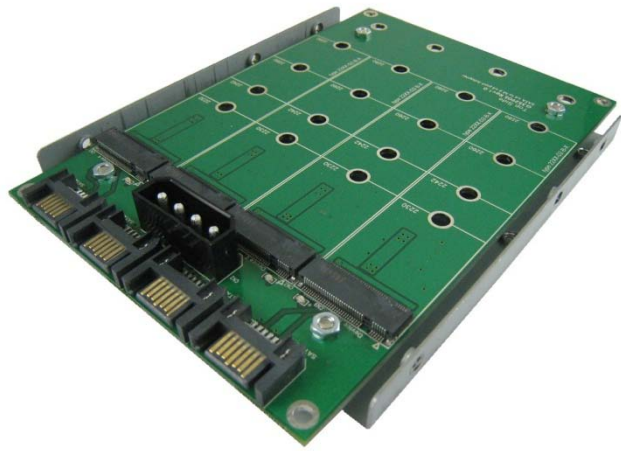
AD904E 转接卡
