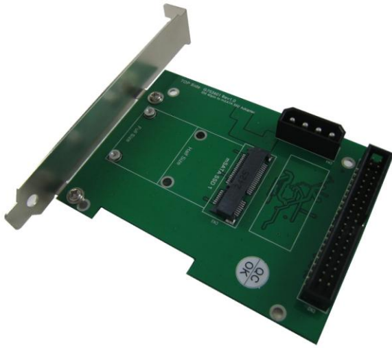
AD263FB9 转接卡 + PCI-e 挡板
